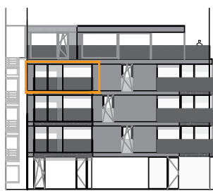
VOORGEVEL NIEUWPOORTSESTEENWEG
