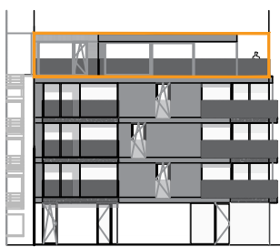
VOORGEVEL NIEUWPOORTSESTEENWEG
